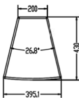
顶视图
